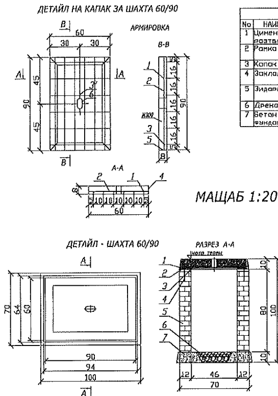
Фиг.6.3. Кабелна шахта – единична
